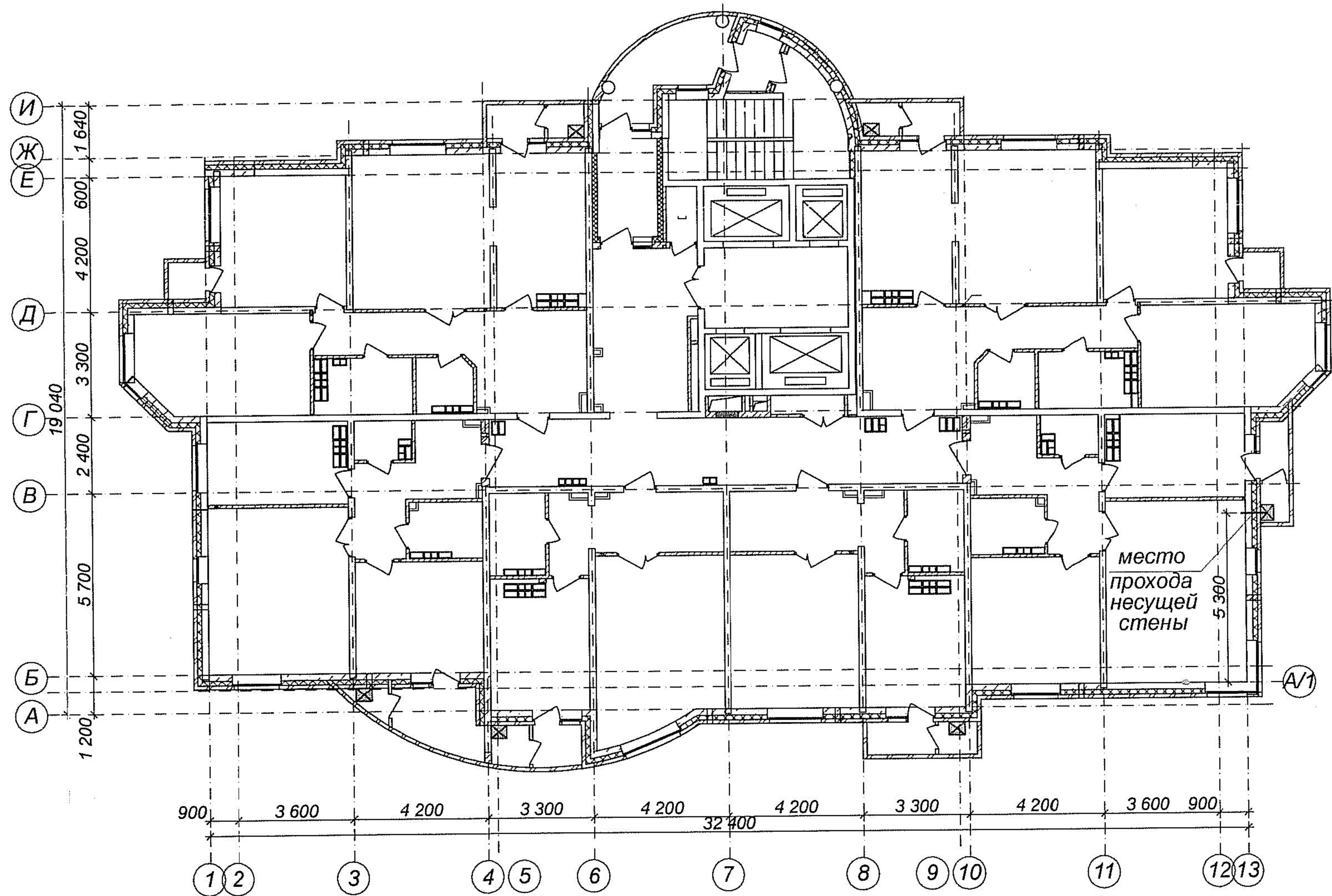
Схема установки кондиционеров на 22...25 этажах
